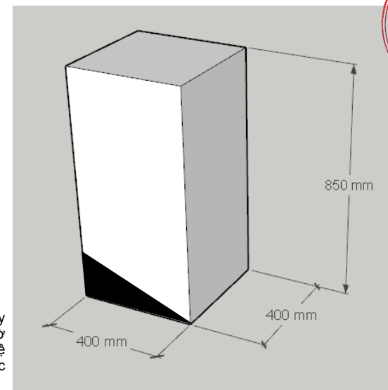
KÍCH THƯỚC CHI TIẾT BỤC N4
