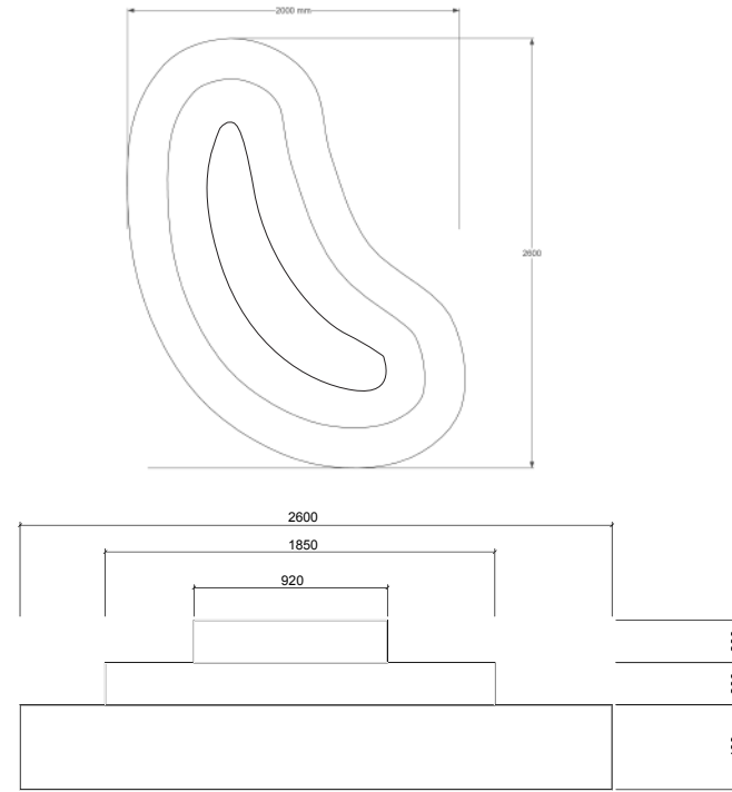
KÍCH THƯỚC BỤC C2
