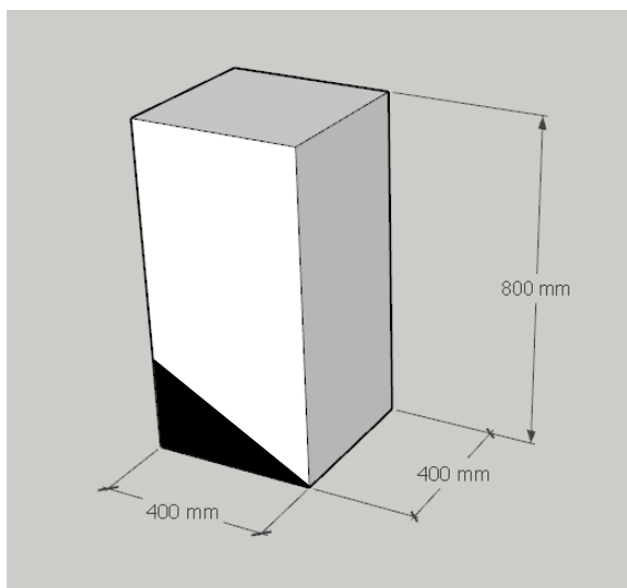
KÍCH THƯỚC CHI TIẾT BỤC N3
