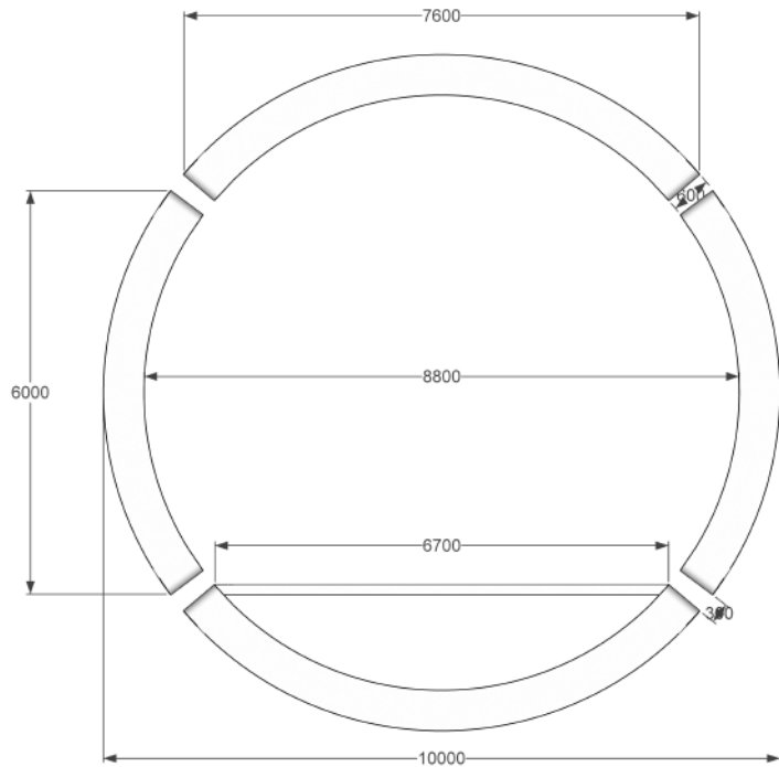
MẶT BẰNG
