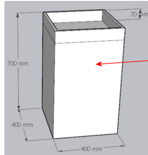
Kích thước bục gỗ
