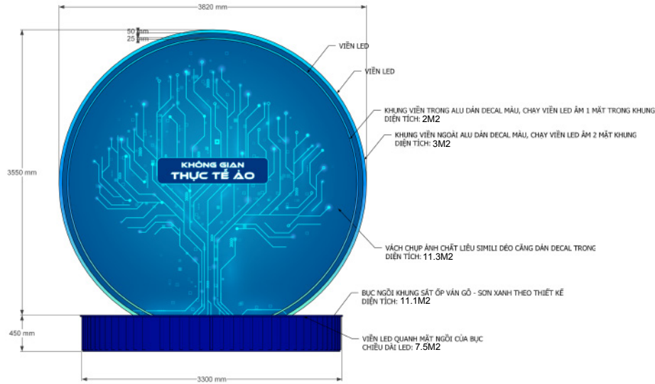
MẶT ĐỨNG
