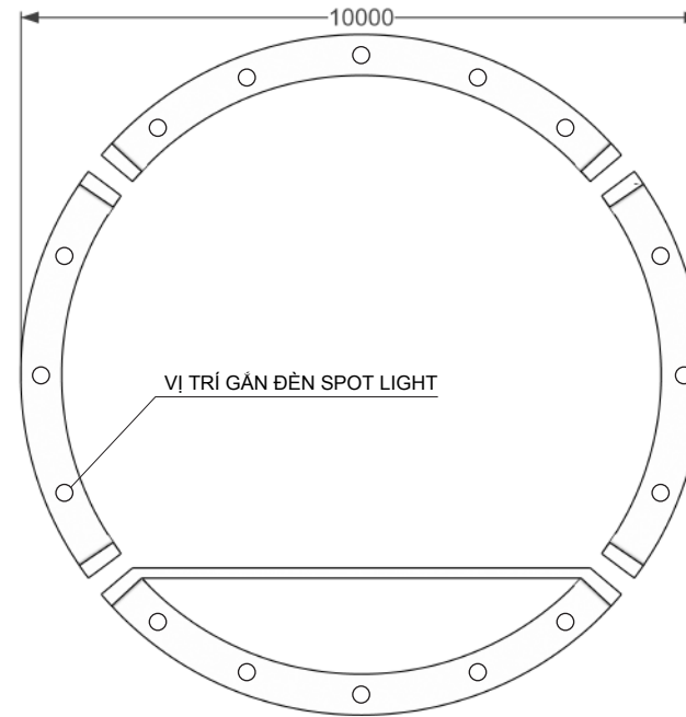
MẶT BẰNG BỐ TRÍ ĐÈN
