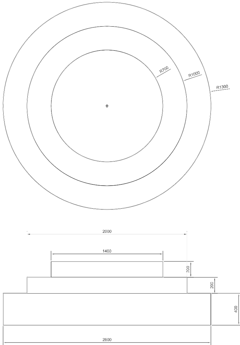
KÍCH THƯỚC BỤC C1
