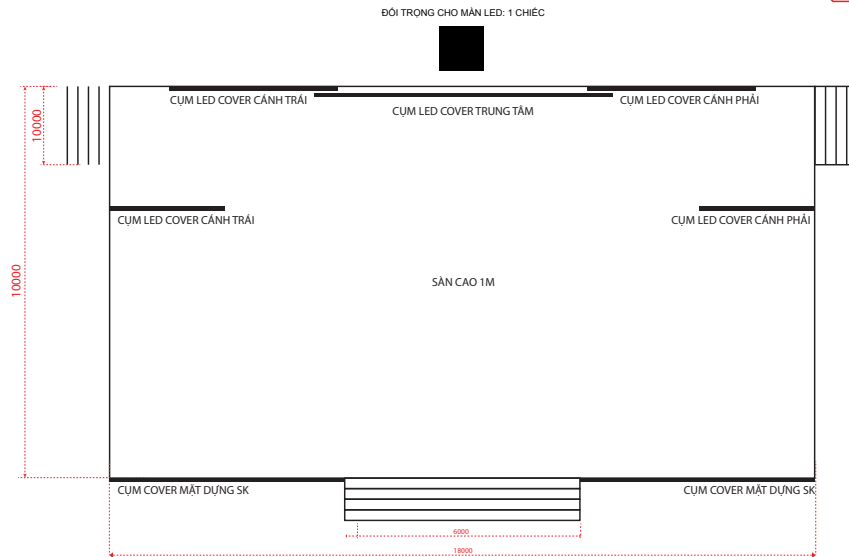
SƠ ĐỒ BỐ TRÍ CÁC HÀNG MỤC TRÊN SÂN KHẤU
