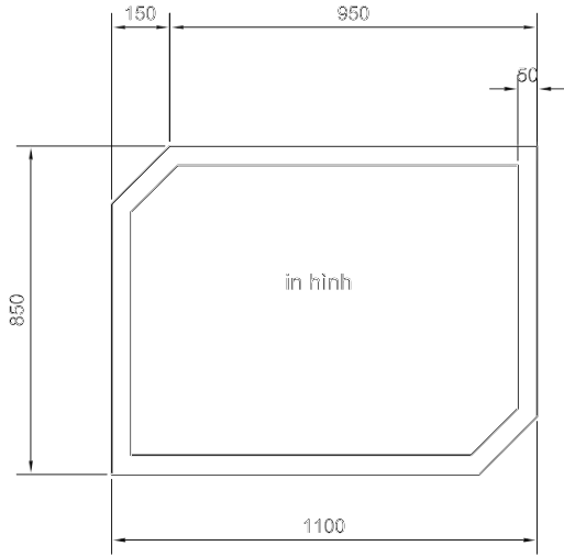
KÍCH THƯỚC BỤC A3
