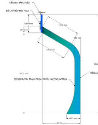
MẶT BÊN
