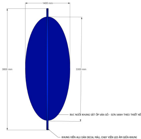
MẶT BẰNG
