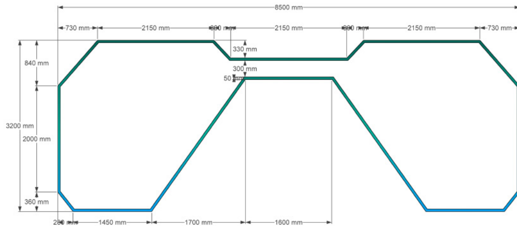
KHUNG ĐỖ VÁCH KÍNH
