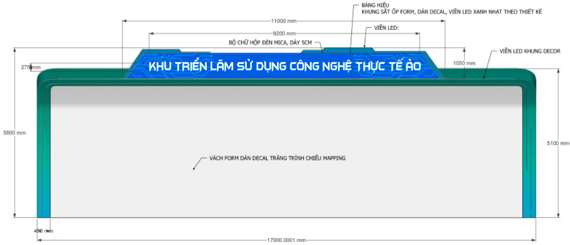
MẶT ĐỨNG
