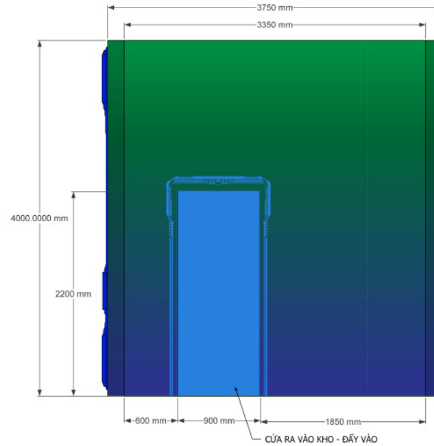
MẶT SAU
