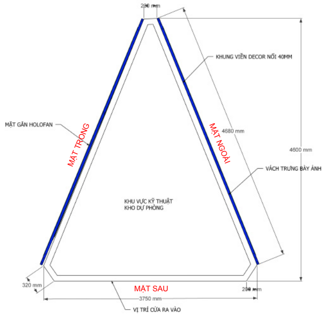
MẶT BẰNG
