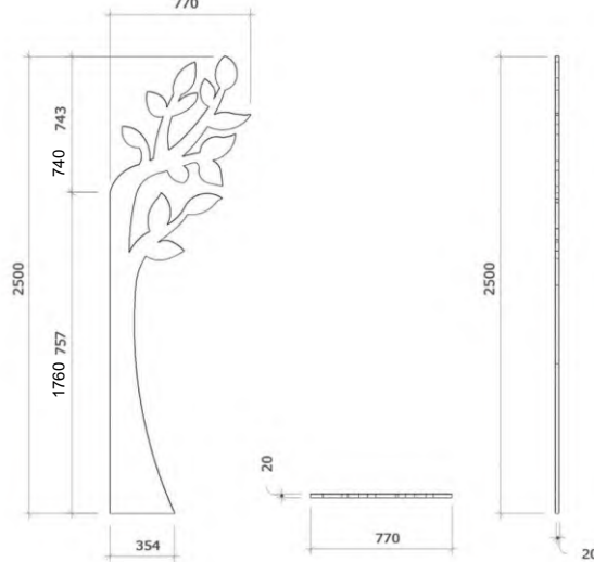
MẶT ĐỨNG
