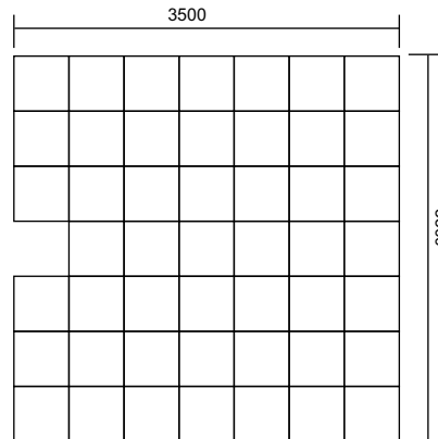
Sơ đồ bố trí ca-bin led: 48 ca-bin 50cm x 50cm (192 module 25cm x 25cm)
