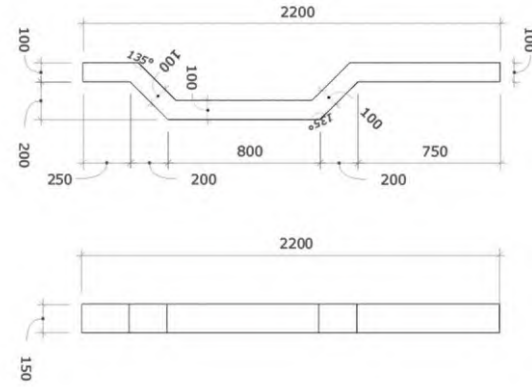
KÍCH THƯỚC CHI TIẾT 8
