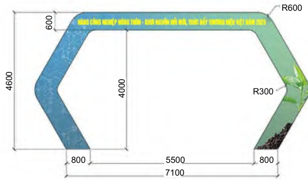
MẶT ĐỪNG CHI TIẾT CÔNG PHỤ (1+2)
