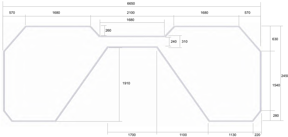
KHUNG ĐỖ VÁCH KÍNH MẶT ĐỨNG
