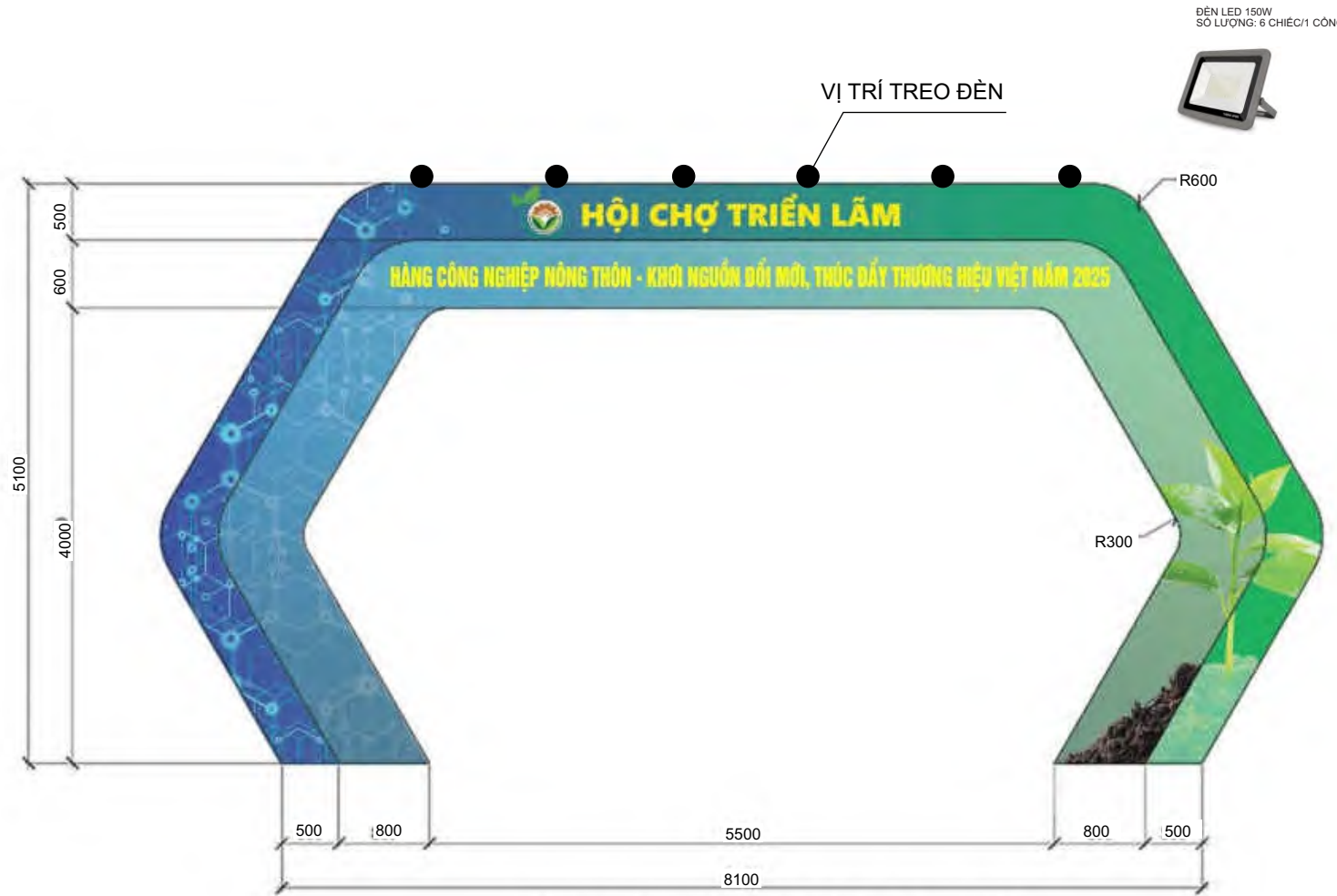
KÍCH THƯỚC CHI TIẾT CÔNG PHỤ (1+2)
