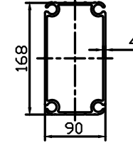
MẶT CẮT CHÂN KÈO
