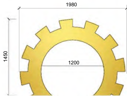
MẶT ĐỪNG MODEL BÁNH RĂNG 1
