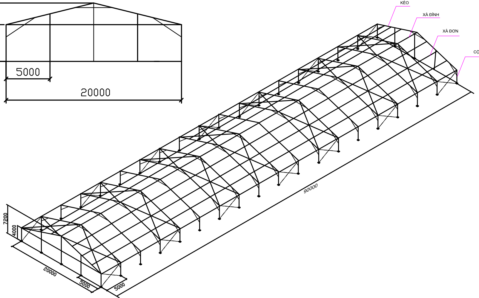
MẶT ĐỨNG 1 VÌ KÈO
