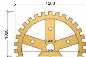
MẶT ĐỪNG MODEL BÁNH RĂNG 2
