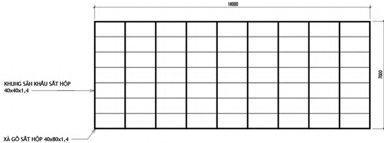
SƠ ĐỒ KHUNG VÀ XÀ GỖ
