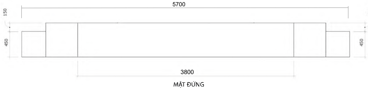
KÍCH THƯỚC BỤC B2
