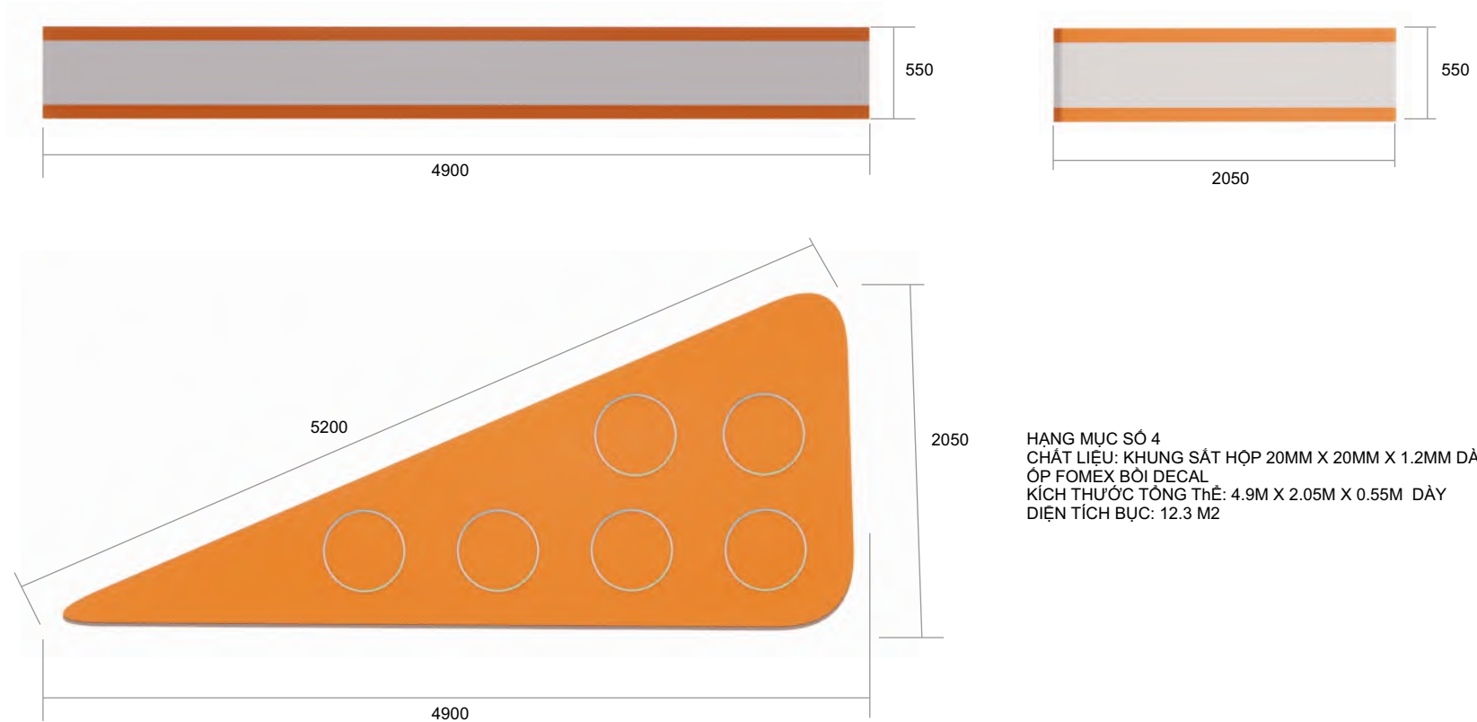
BỤC TAM GIÁC TRƯNG BÀY SẢN PHẨM
