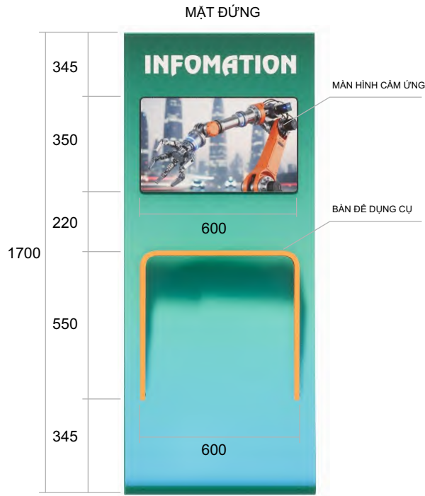
BỤC ĐỀ MÁY CHIẾU (MAPPING)
