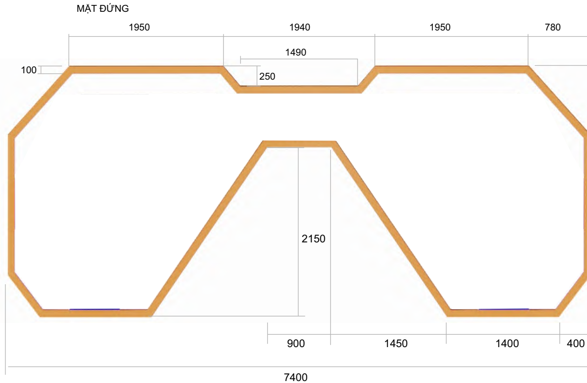
KHUNG VÁCH CÔNG BÊN TRÁI
