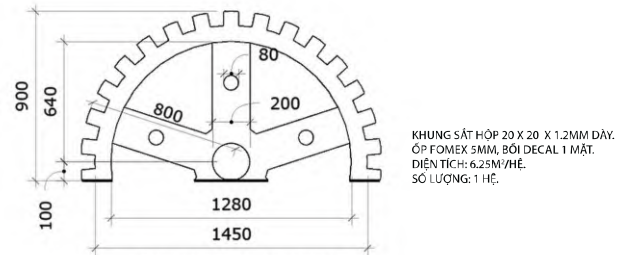
BÁNH RĂNG 6 - DÀY 200
