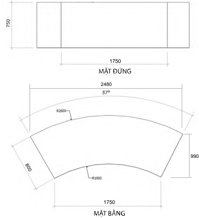
KÍCH THƯỚC BỤC A2
