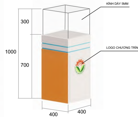
BỤC TRƯNG BÀY SẢN PHẨM NHỎ
