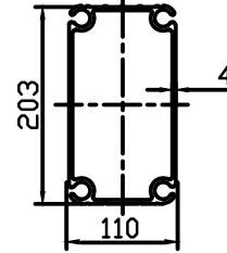
MẶT CẮT CHÂN CỘT
