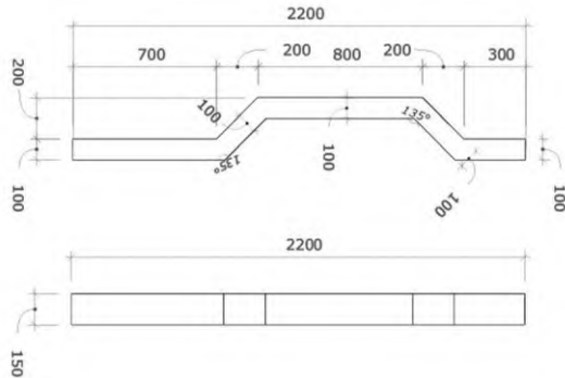
KÍCH THƯỚC CHI TIẾT 9
