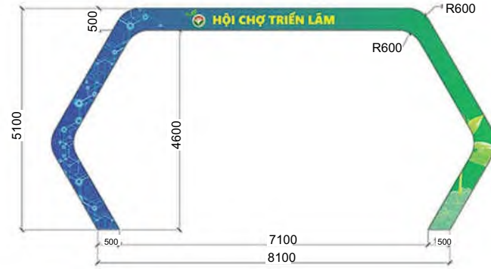
MẶT ĐỪNG CHI TIẾT CÔNG PHỤ (1+2)
