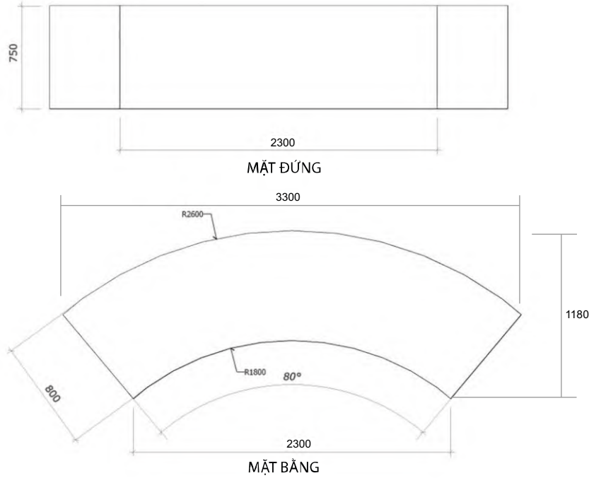
KÍCH THƯỚC BỤC A1
