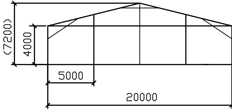
MẶT ĐỨNG 1 VÌ KÈO
