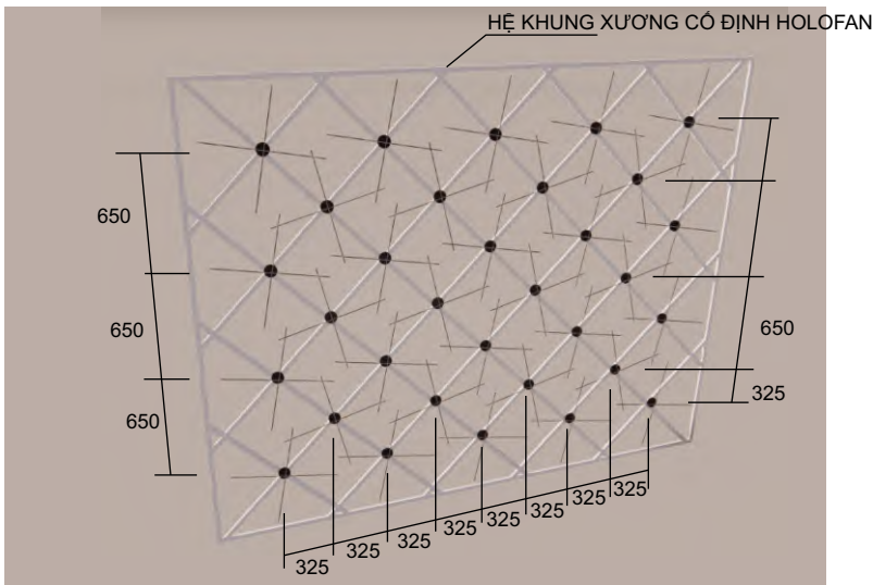
VỊ TRÍ TREO QUẠT HOLOFAN
