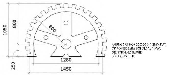
BÁNH RĂNG 2 - DÀY 200
