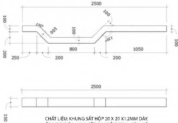
KÍCH THƯỚC CHI TIẾT 6
