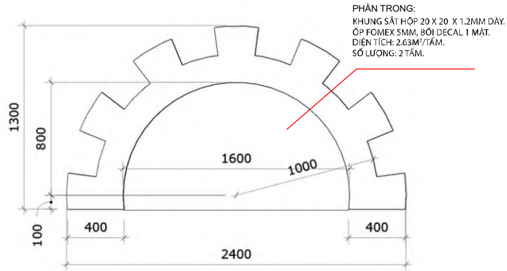
BÁNH RĂNG 1 - DÀY 150
