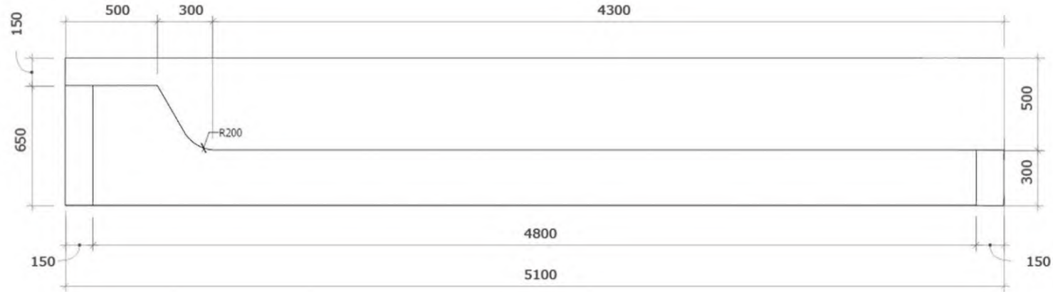
KÍCH THƯỚC CHI TIẾT 5
