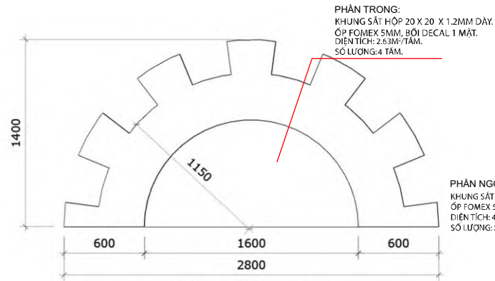
BÁNH RĂNG 4 VÀ 5 - DÀY 150
