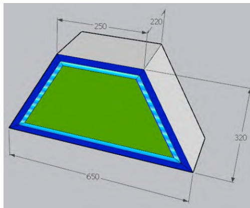
GIÁ ĐỖ VÁCH KÍNH
