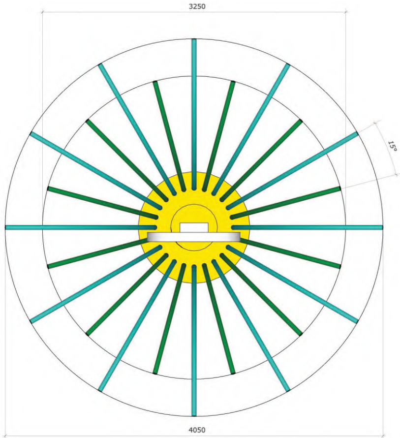
MẶT BẰNG
