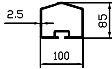
MẶT CẮT XÀ ĐÌNH
