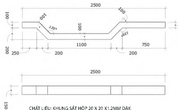
KÍCH THƯỚC CHI TIẾT 10
